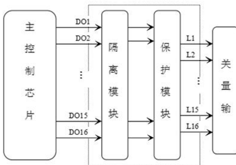
图 4-3-3-1 DO710 原理图
