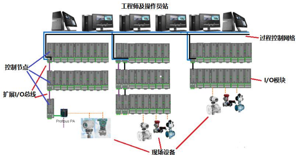
图 1-2 系统结构
