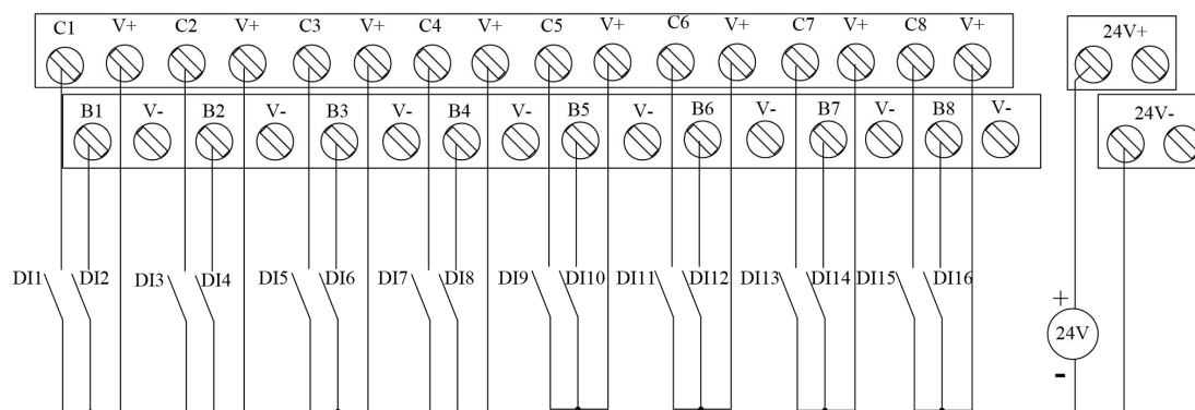
图 4-3-1-2 DI710 接线示意图
