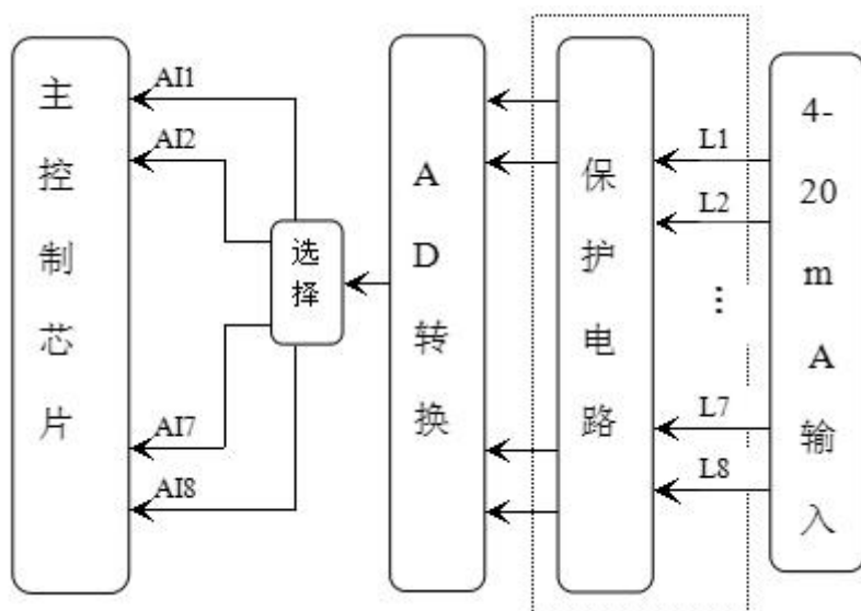
图 4-3-4-1 AI710 原理图
