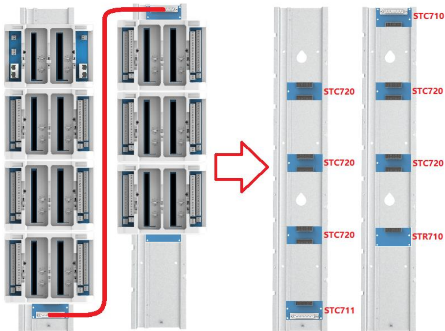
图 5-4-1-3 导轨配件安装配置图 2
