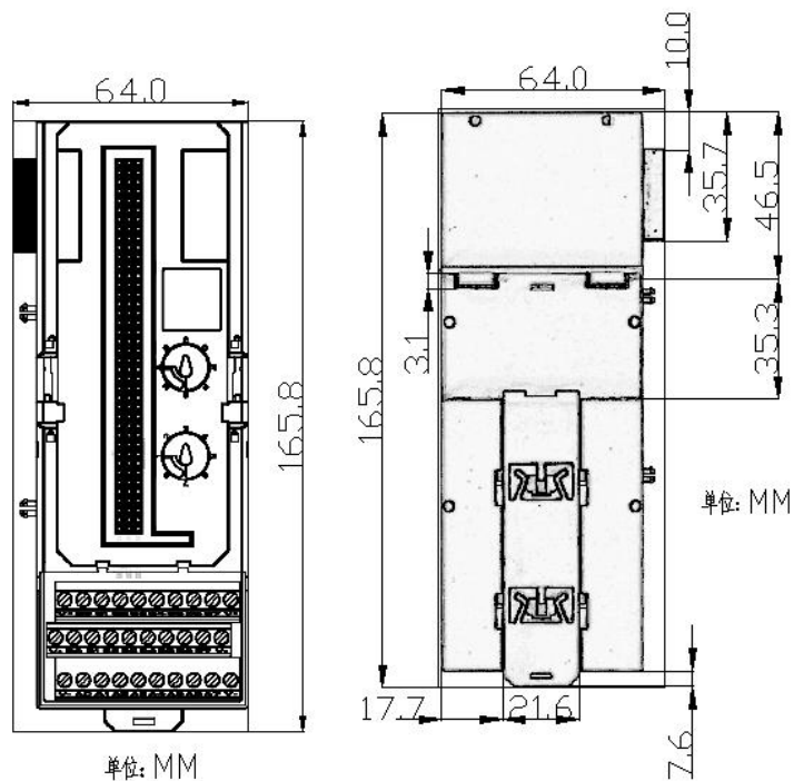
图 5-2-1-1 TU710 接线端子式 IO 模块底座尺寸图
