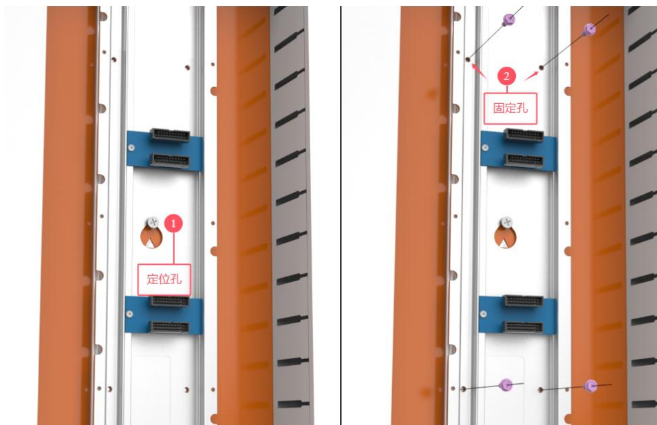
图 5-4-2-2 导轨固定安装示意图
