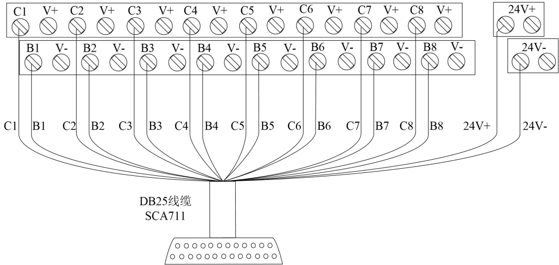
图 4-3-3-4 DO710 端子接线图
