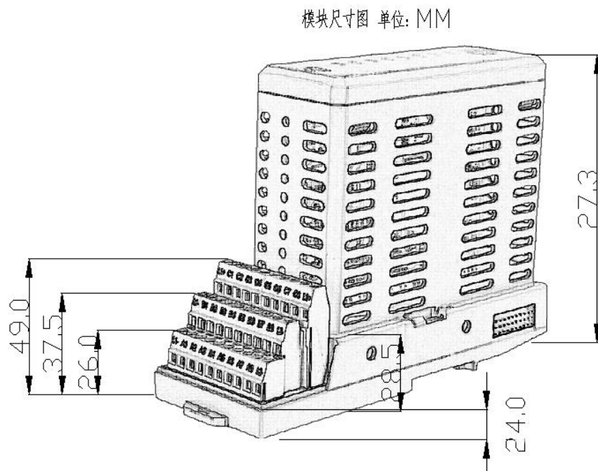
图 5-2-2-1 整体模块尺寸图
