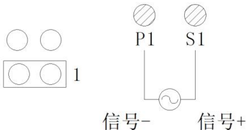
图 4-5-7-3 模拟量输出接线示意图
