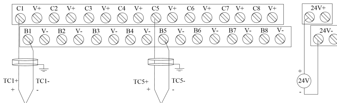
AI740-STU710底座外部接线图
