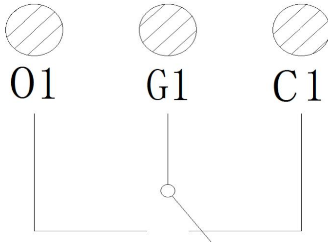
图 4-5-2-1 D0T710 接线示意图
