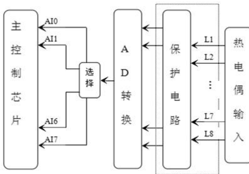
图 4-3-6-1 AI740 原理图
