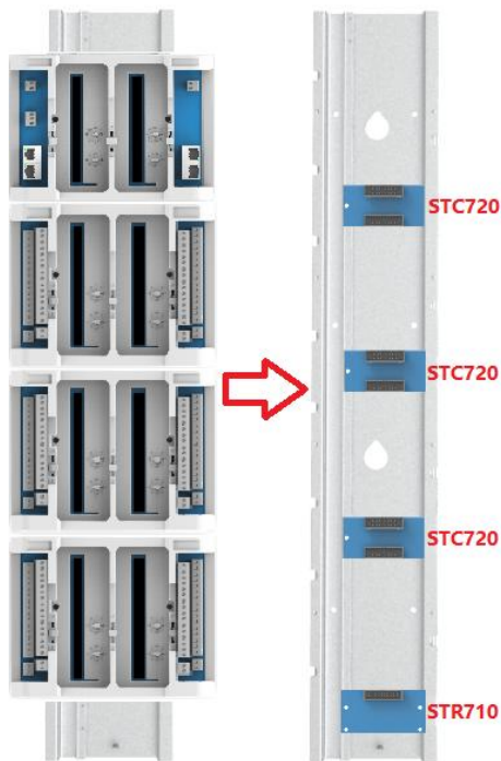
图 5-4-1-4 导轨配件安装配置图 3
