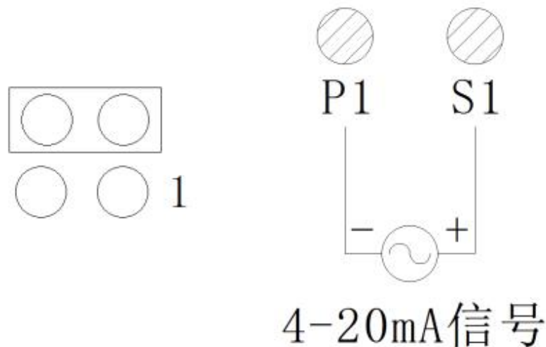
图 4-5-7-2 四线制接线示意图
