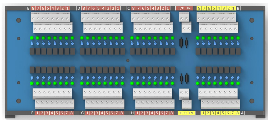
图 4-5-8-1 模拟量输出接线示意图
