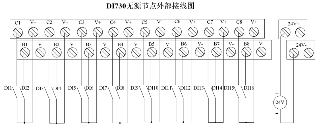
图 4-3-2-2 DI730 接线示意图
