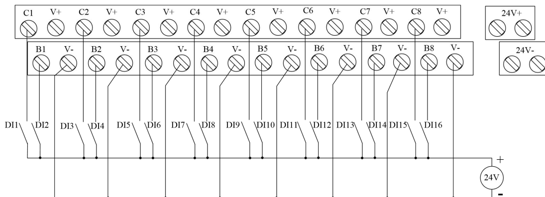
图 4-3-2-3 DI730 接线示意图
