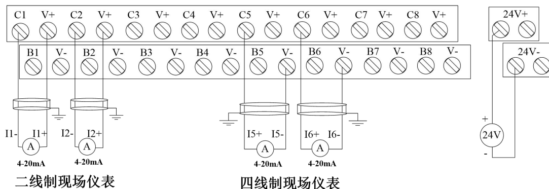
AI710-STU710底座外部接线图
