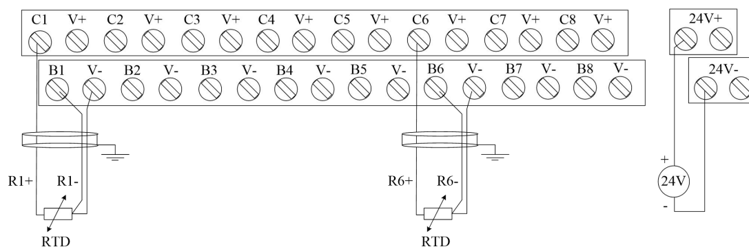
AI730-STU710底座外部接线图
