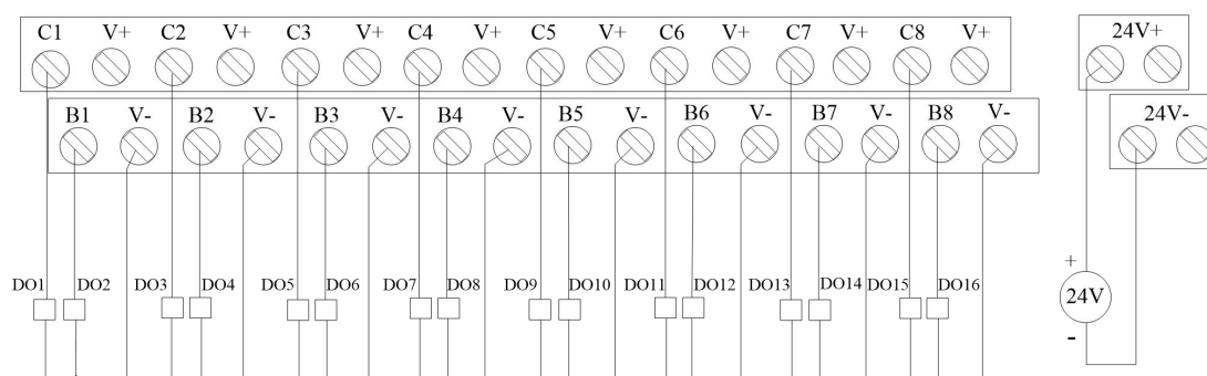
DO710-STU710底座直连外部接线图
