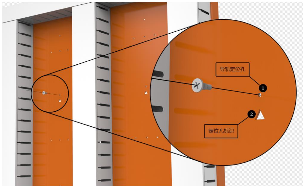
图 5-4-2-1 导轨定位孔螺丝安装示意图
