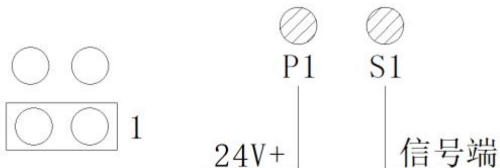
图 4-5-7-1 二线制接线示意图
