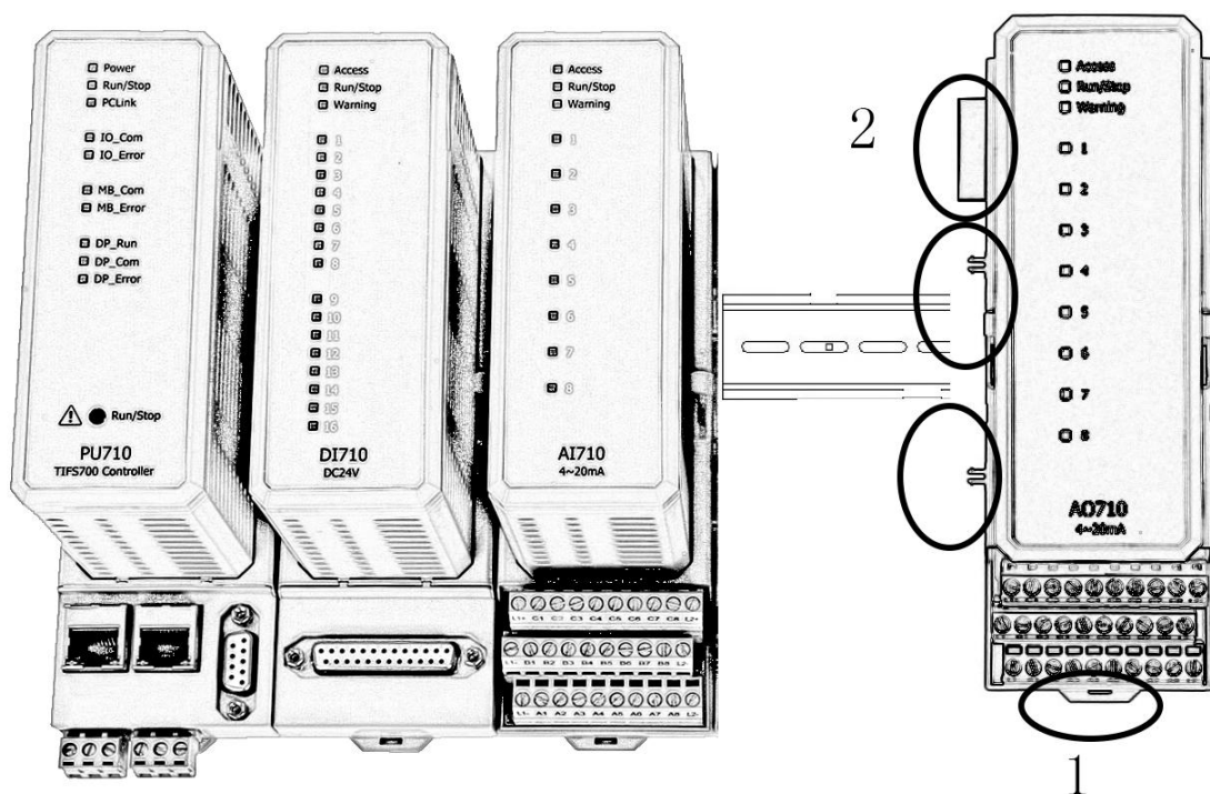
图 5-3-2-1 底座与导轨安装图
