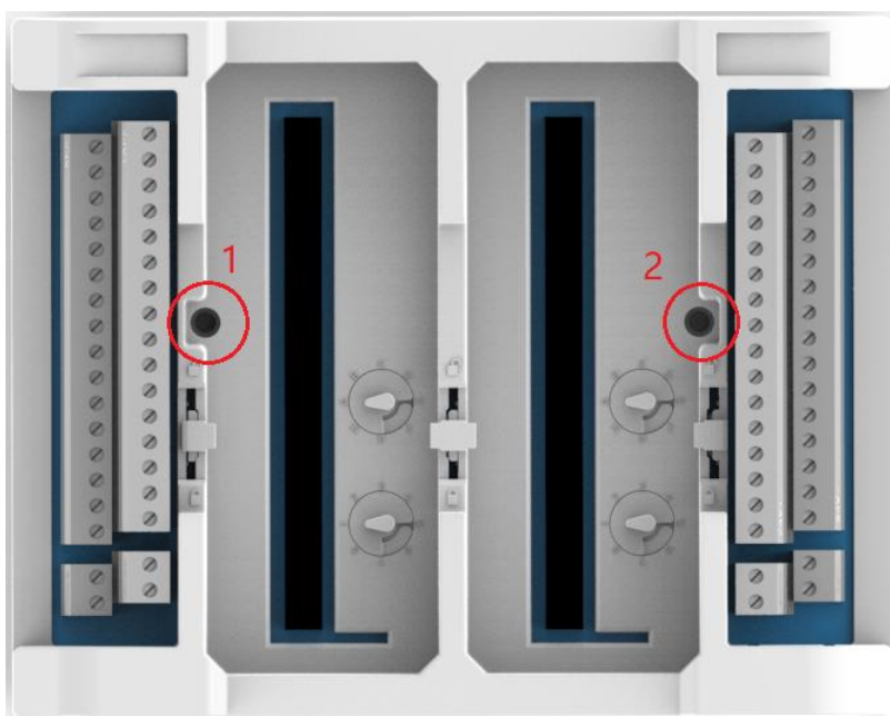
图 5-4-3-2 底座固定示意图
