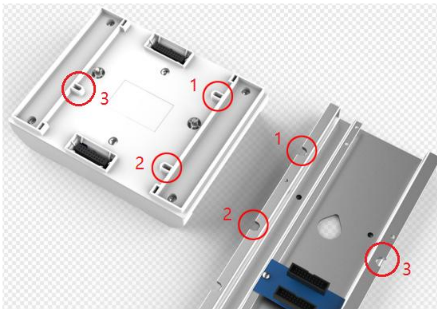
图 5-4-3-1 底座安装示意图
