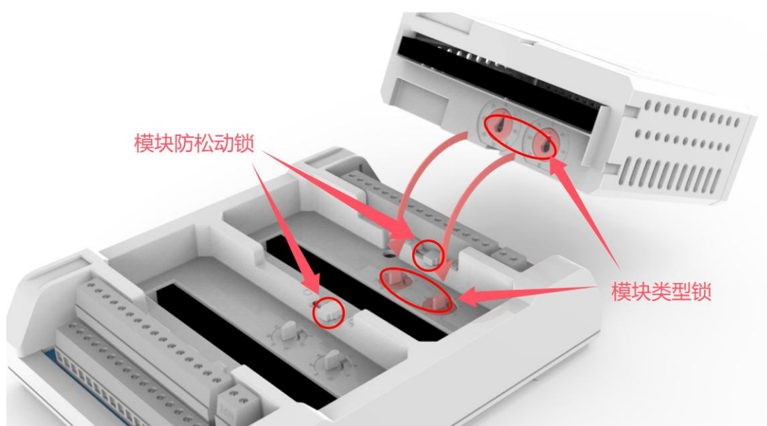
图 5-4-4-1 模块安装示意图
