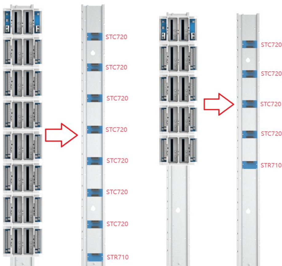
图 5-4-1-2 导轨配件安装配置图 1
