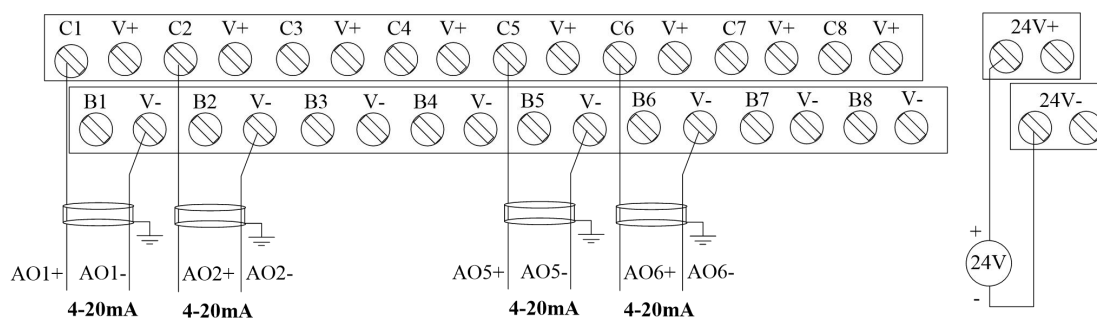
图 4-3-7-2 AO710 端子接线图
