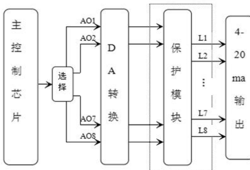
图 4-3-7-1 AO710 原理图
